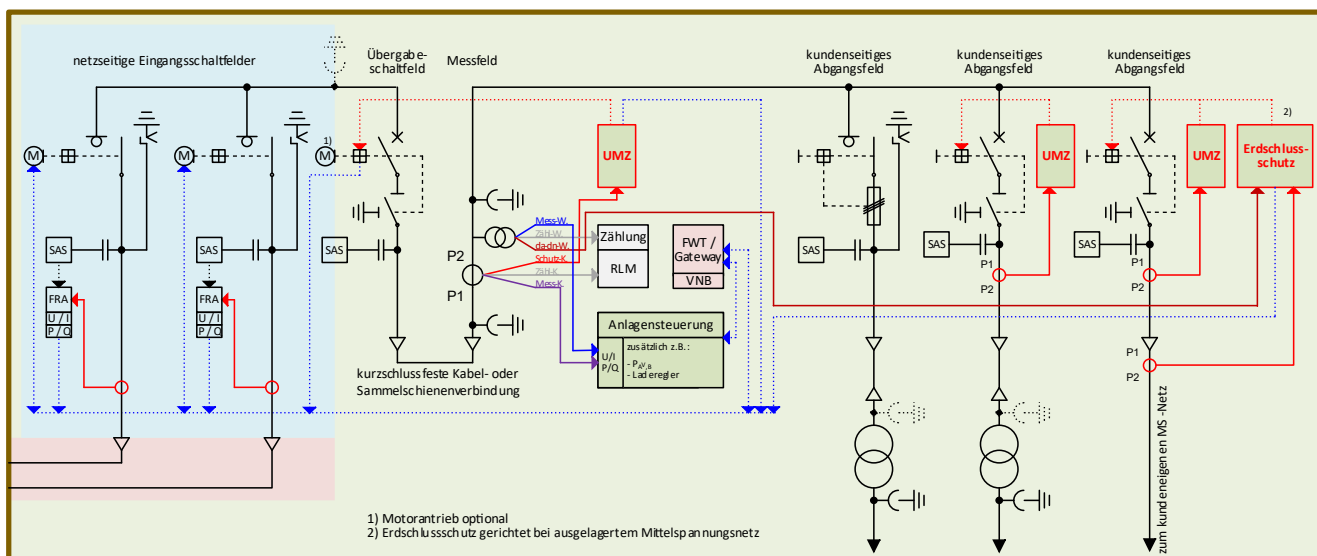
Bild D.3 Ergänzung zu Bild D2 (K)K-LM-TLL des BDEW-Musterwortlauts [7]: MS-Bezugsanlage – Übergabeschalter als Leistungsschalter , mehrere kundenseitigen Abgangs- bzw. Transformatorenfelder und kundenseitig betriebenes MS-Netz
